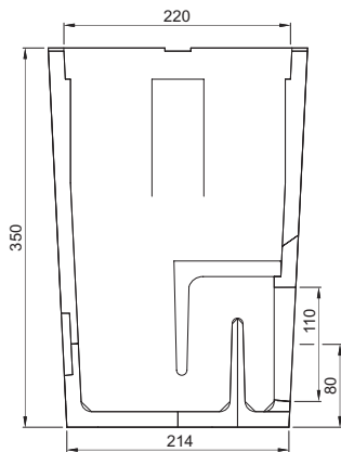
Secțiune A-A
