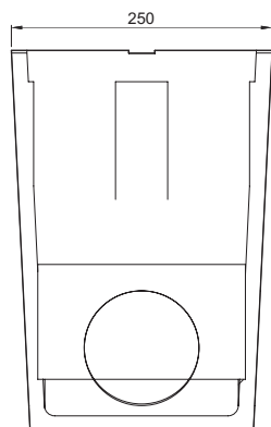
Secțiune B-B
