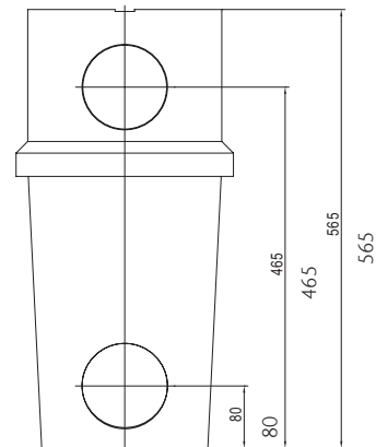
Cu element de înălțare
