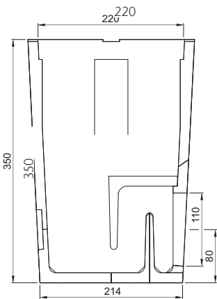
Secțiune A-A
